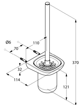
RYSUNEK Z WYMIARAMI
