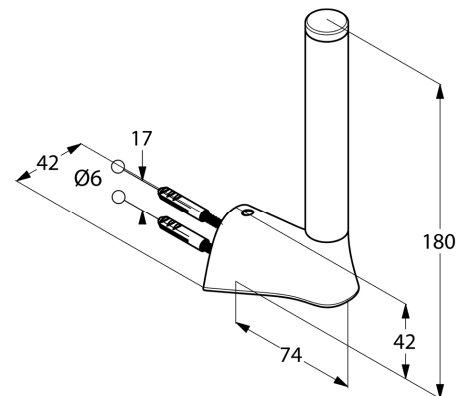
RYSUNEK Z WYMIARAMI
