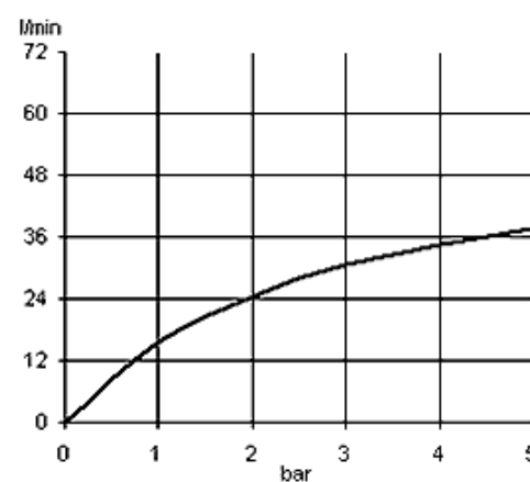
Diagram przepływu
