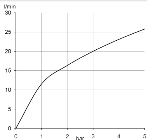
DIAGRAM PRZEPEŁYWU
