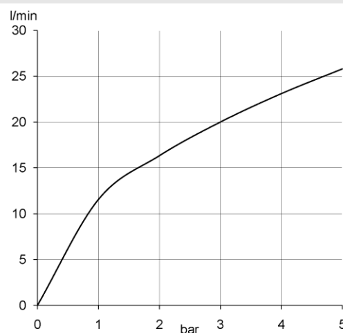
DIAGRAM PRZEPEŁYWU
