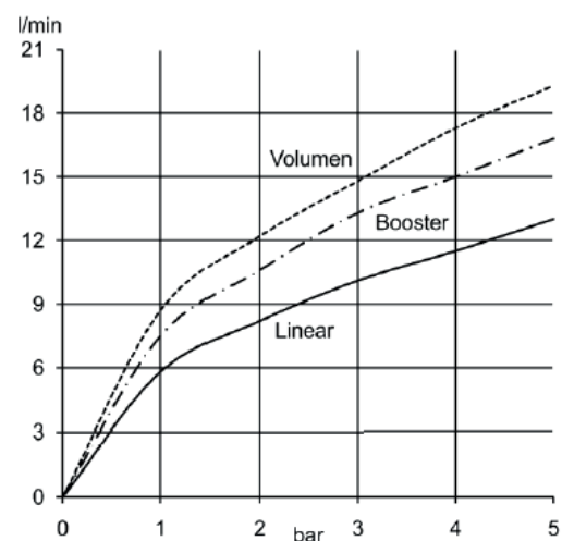
Diagram przepływu
