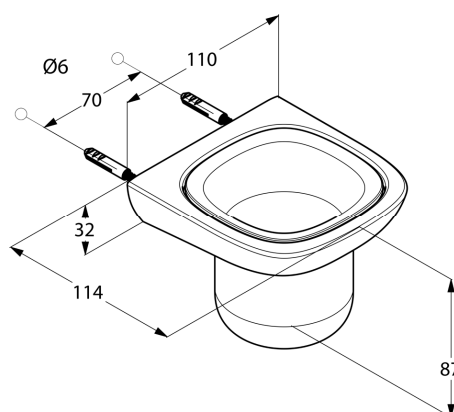
RYSUNEK Z WYMIARAMI
