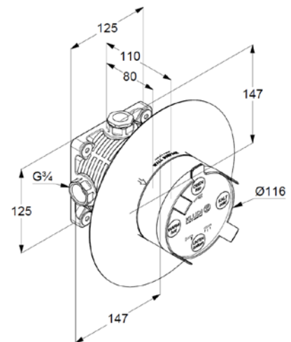
RYСУNEK Z WYMIARAMI
